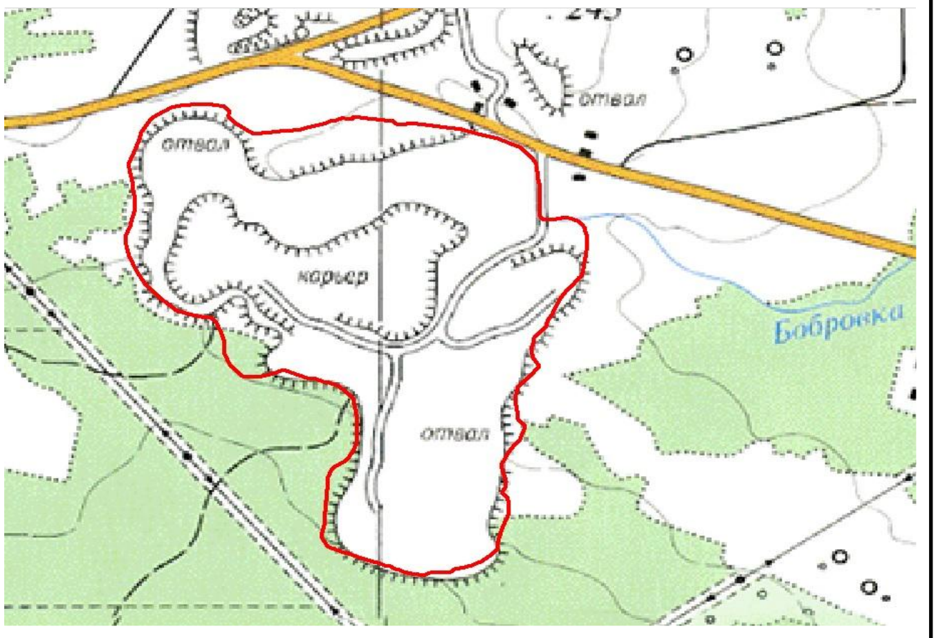
Границы большого Липовского карьера.
